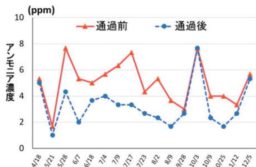
図2 養鶏農家におけるアンモニア濃度の推移
