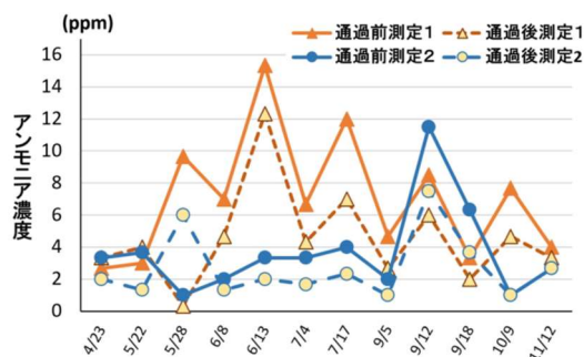
図3 養豚農家におけるアンモニア濃度の推移
